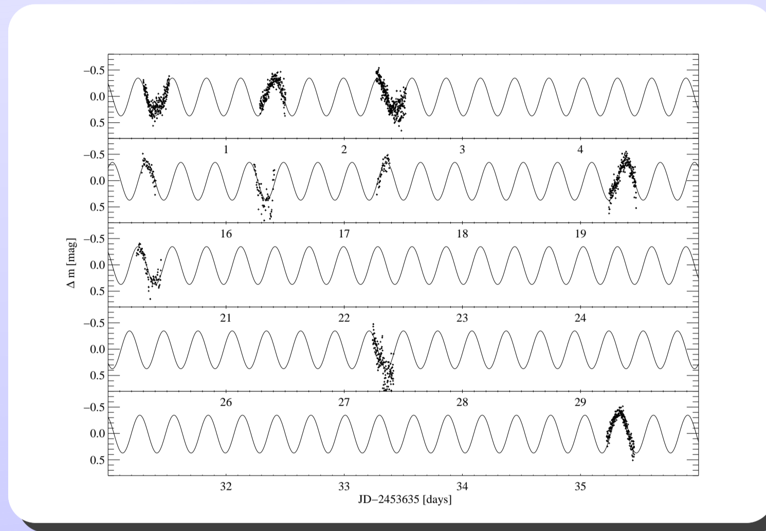
ABB. 2: Lichtkurve von SDSS J212531.92-010745.9 für 10 Beobachtungsnächte im September und Oktober 2005. Darübergezeichnet ist eine Sinuskurve mit einer Periode von 6.95616(33) h.
