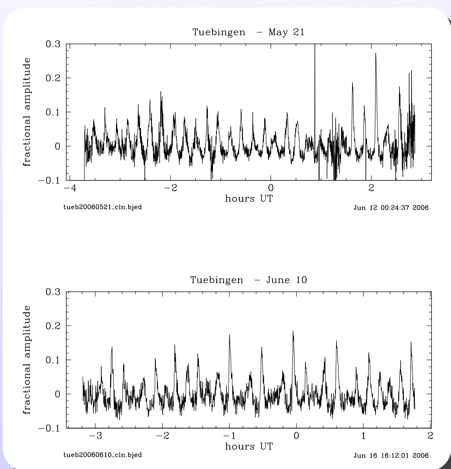
ABB. 6: Lichtkurven von GD 358 am 21.5. und 6.10.2006.
