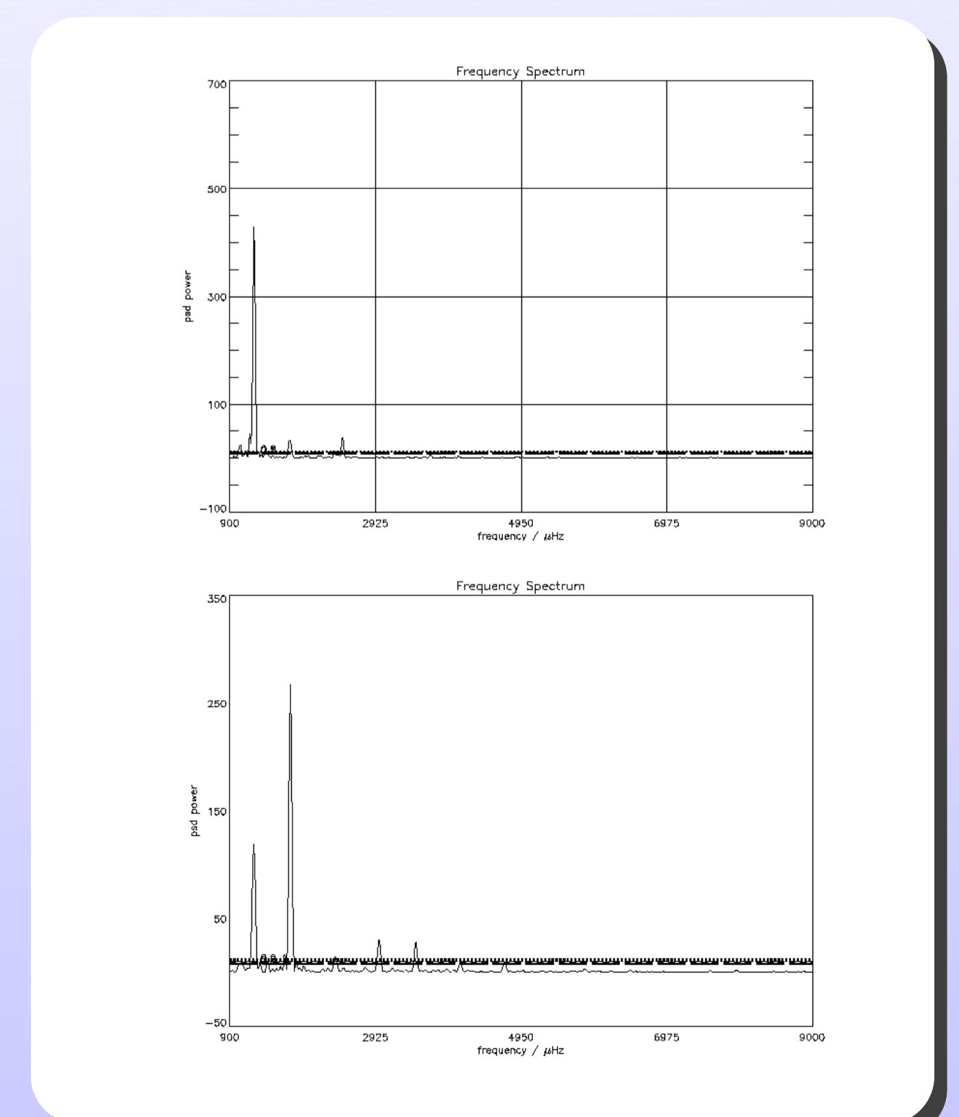
ABB. 7: Periodogramme zu den Lichtkurven von GD 358.
