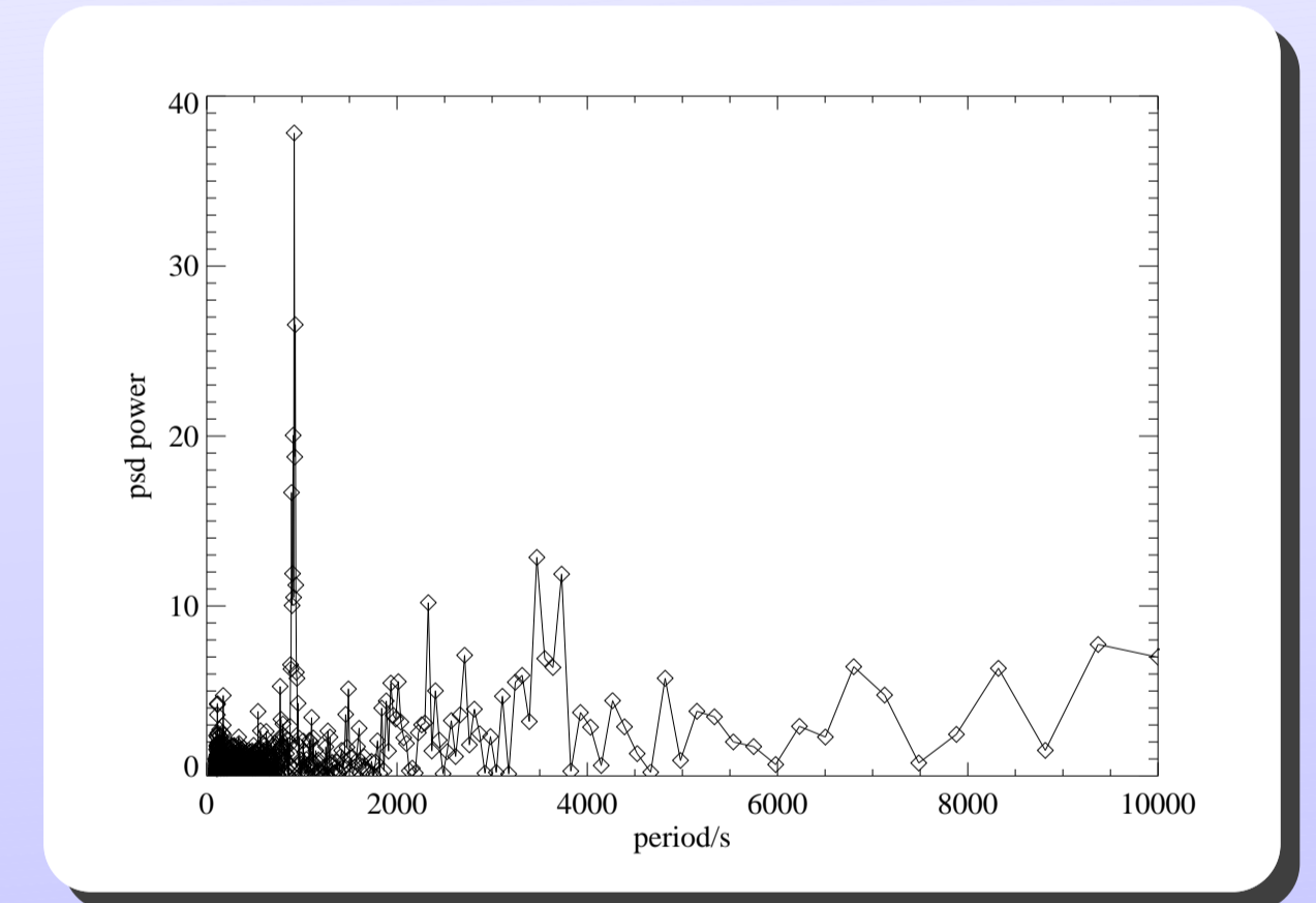
ABB. 5: Periodogramm zur Lichtkurve von HE 1429-1209. Die gefundene Pulsationsperiode von 919 s ergibt sich aus dem höchsten Peak, die Grenze für 99% Wahrscheinlichkeit liegt bei 11,8.
