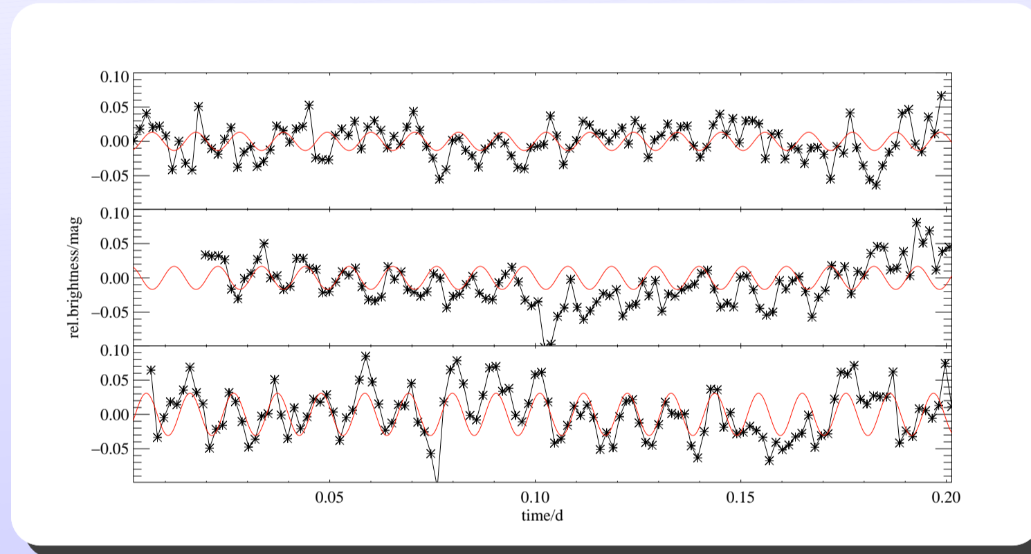
ABB. 4: Lichtkurve von HE 1429-1209. Darübergezeichnet ist eine Sinuskurve mit der von uns bestimmten Periode von 919 s.
