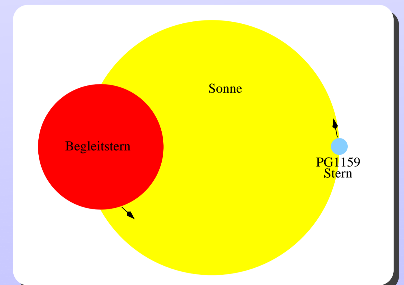
ABB. 3: Größenvergleich des entdeckten Doppelsterns mit unserer Sonne.
