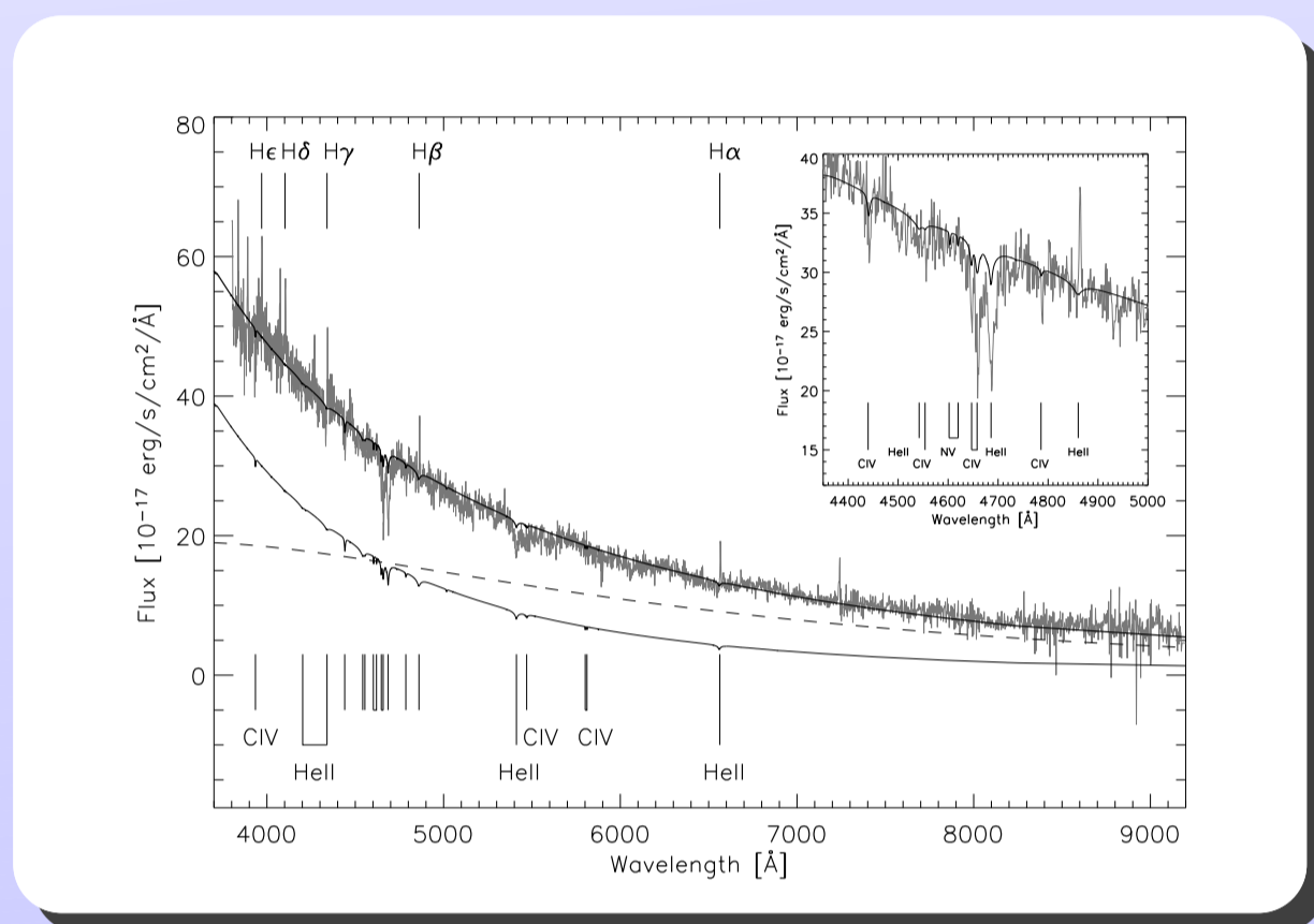
ABB. 1: Spektrum von SDSS J212531.92-010745.9 und ein berechnetes Modellspektrum zum Vergleich. Einige auffällige Spektrallinien sind markiert.
